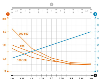
Belastungsdiagramm Gitterrinne Typ GRM 105
